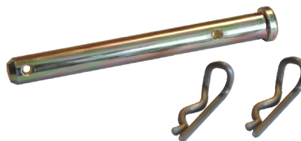
L3528110 oś zacisku hamulcowego 55 mm 29,80 zł L3528120 oś zacisku hamulcowego 60 mm 29,80 zł
