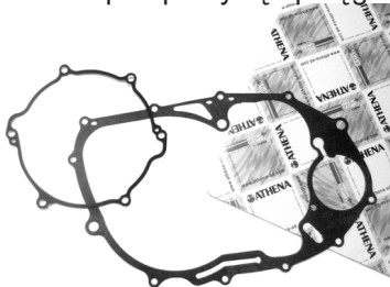
uszczelki pod pokrywę sprzęgła*
